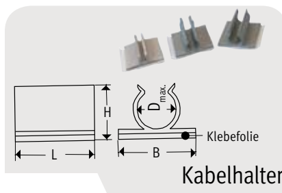
Kabelhalter
