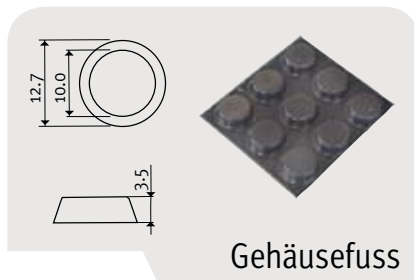
Gehäusefuss
