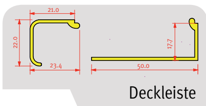
Deckleiste
