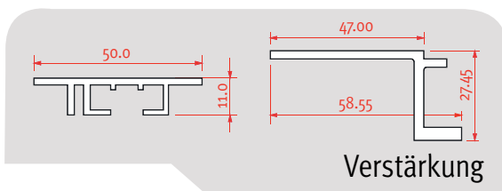
Deckleiste
